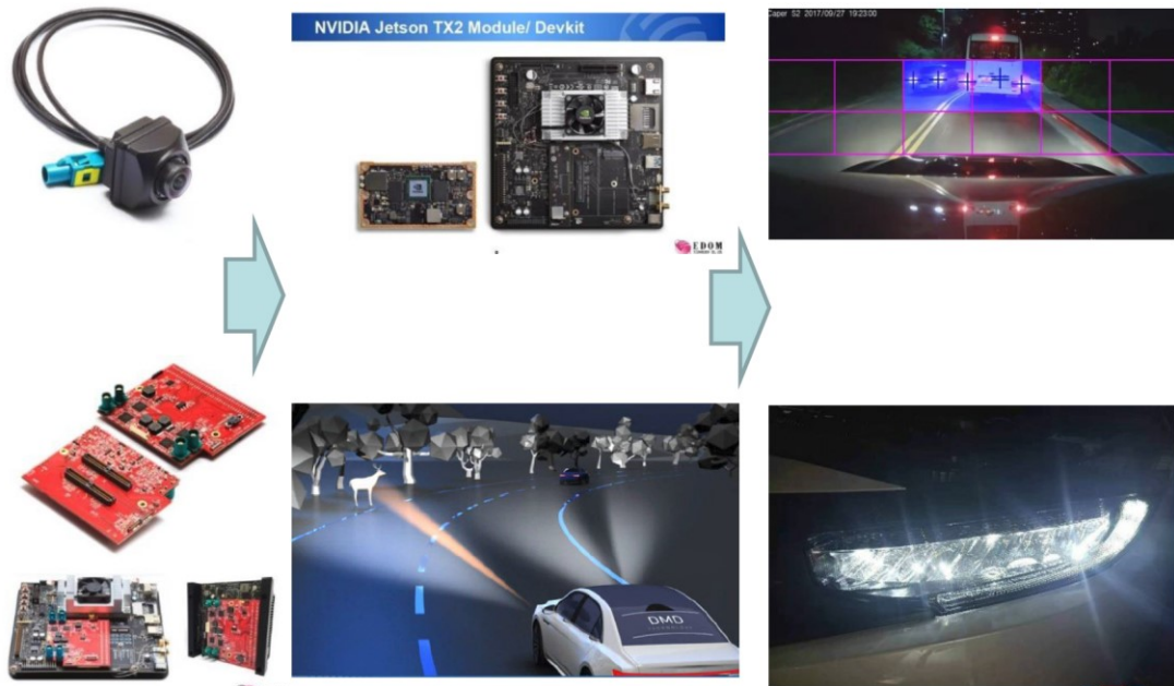
智慧車燈系統與設備整合示意圖
